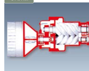
联轴器
